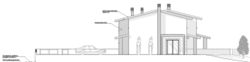
Prospetto Laterale Ovest
